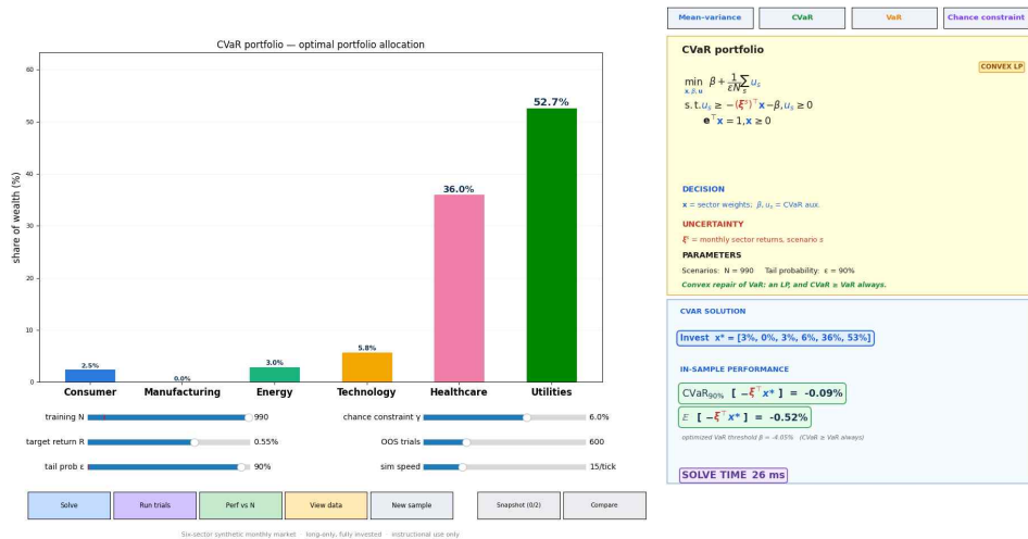
그림 1. CVaR·VaR·확률제약(Chance constraint) 기반 포트폴리오 최적화(4·6주차)
